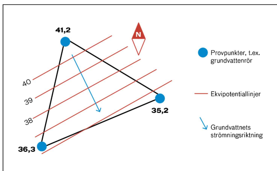
Figur 1 Grundvattnets strömningsriktning kan bestämmas med en så kallad "hydraulisk triangel" där nivåerna mäts i tre punkter. Strömningsriktningen (den blå pilen) ligger vinkelrätt mot ekvipotentiallinjerna (de röda linjerna).
