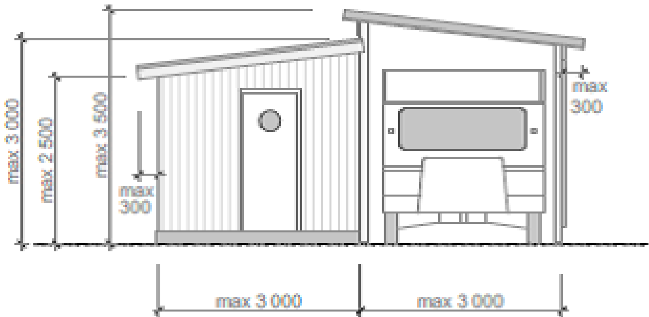
Fasad framsida med infart, fasad 2 - 1:100
