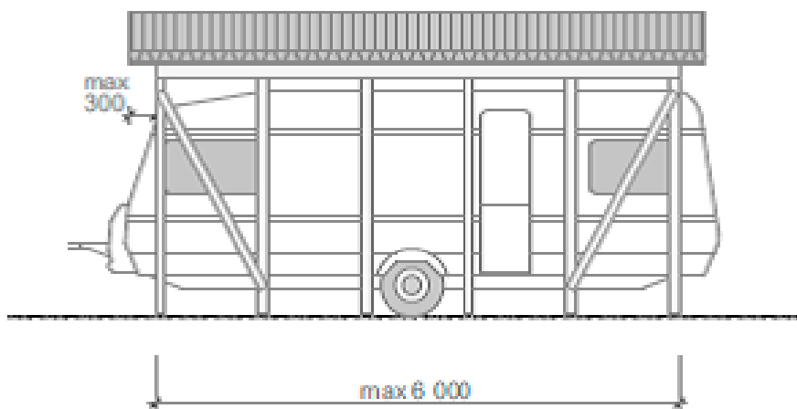
Fasad sida skärmtak, fasad 3 - 1:100
