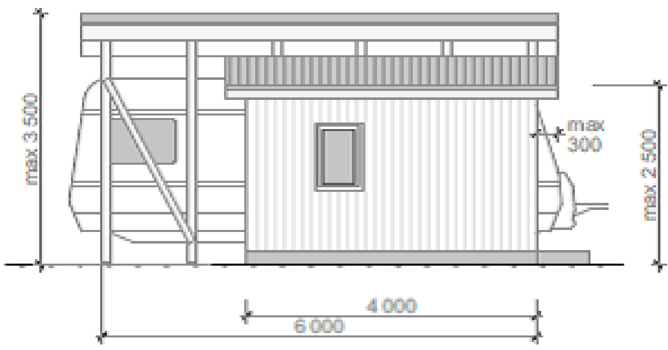
Fasad sida spiketält, fasad 1 - 1:100
