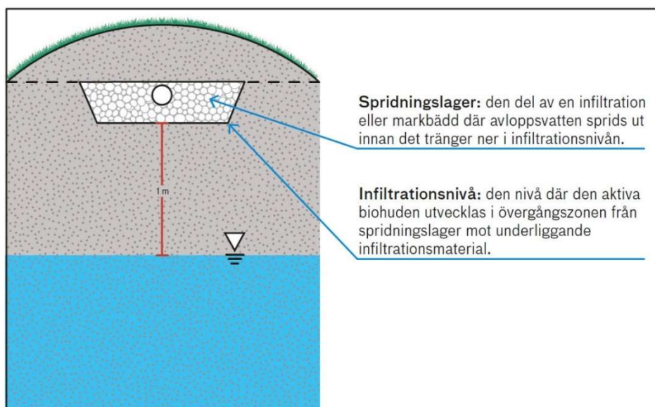
Figur 1 För att reningen i en infiltrationsanläggning ska fungera ska avståndet mellan infiltrationsnivån och den högsta dimensionerande grundvattennivån (den omättade zonen) vara minst 1 meter under större delen av året.
