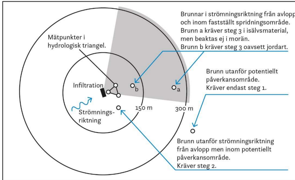
Figur 2 Principskiss över utredningsmodell med exempel på brunnpositioner. Figuren illustrerar gränser för potentiellt påverkansområde i morän (den lilla cirkeln) och isälvsmaterial (den stora cirkeln) samt fastställt spridningsområde (det grå fältet). Vinkeln på det grå fältet kan variera. Med en flackare terräng och därmed svag gradient på grundvattnets lutning, blir spridningen bredare och spridningsriktningen mer ovisst.
