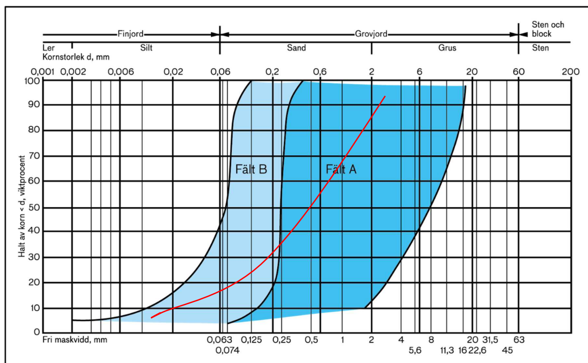
Figur 5 Resultat av siktanalys
