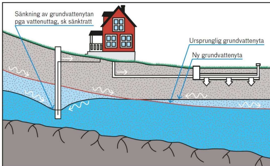
Figur 4 Vattentäkt och avloppsanläggning kan ändra grundvattnets strömningsriktning.
