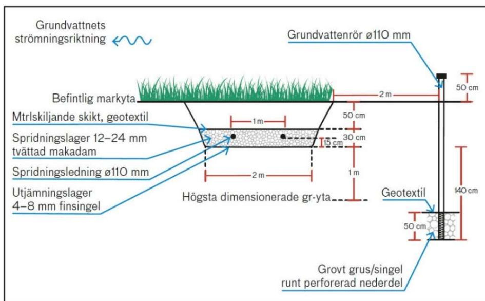
Figur 2 Exempel på tvärsektionsritning över infiltration med grundvattenrör för kontroll av grundvattennivå. Rörets botten bör ligga minst 140 cm under infiltrationsnivån (undre kanten på spridningslagret i detta exempel). Bifoga en tvärsektionsritning som underlag för installationsarbetet till din ansökan.
