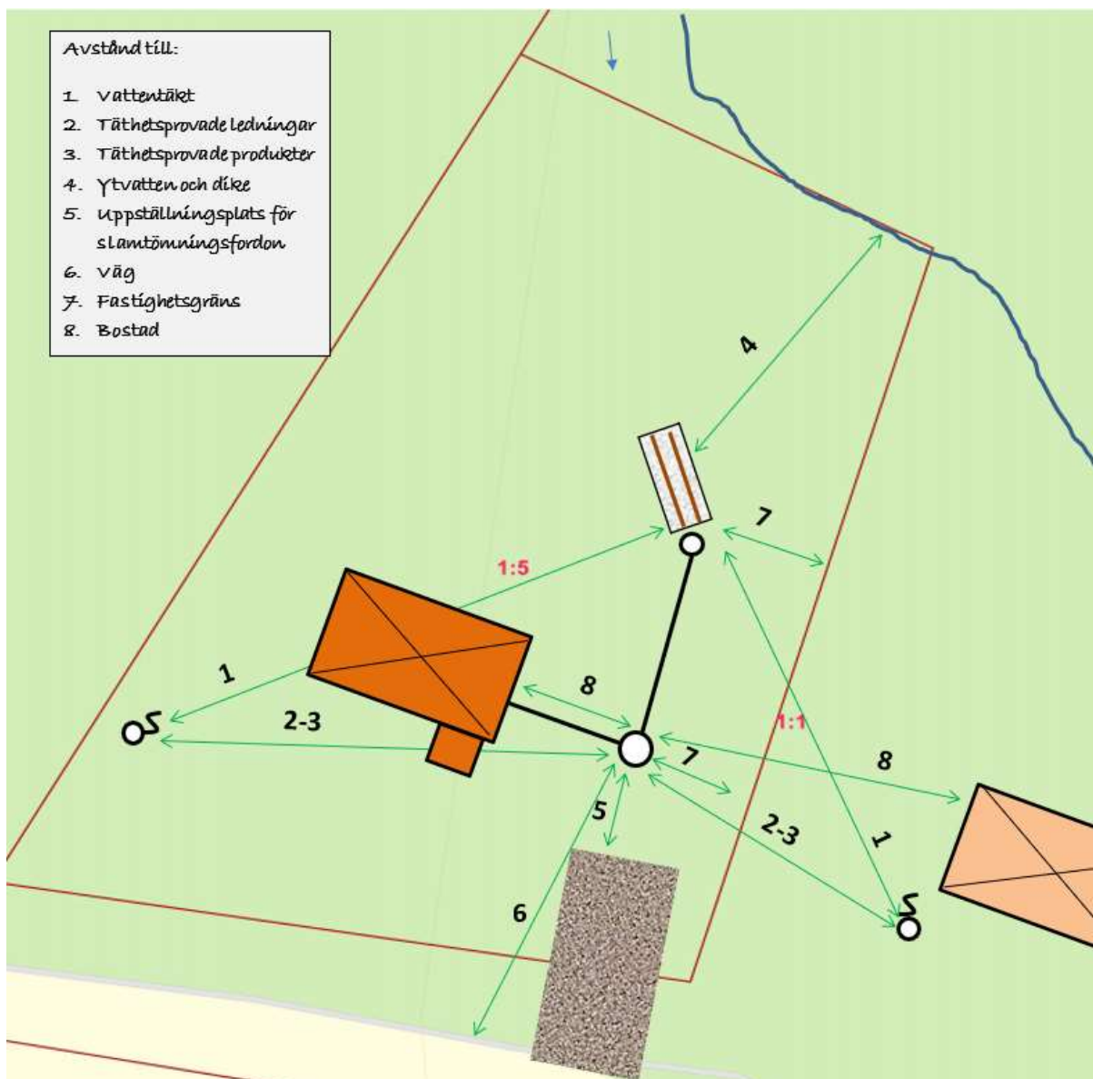
Figur 2 Horisontella skyddsavstånd
